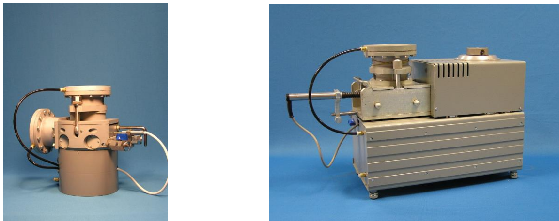
Рис. 1. Приборы для испытаний грунтов в условиях одноплоскостного среза
